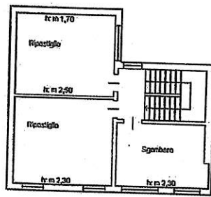
Piano terzo
